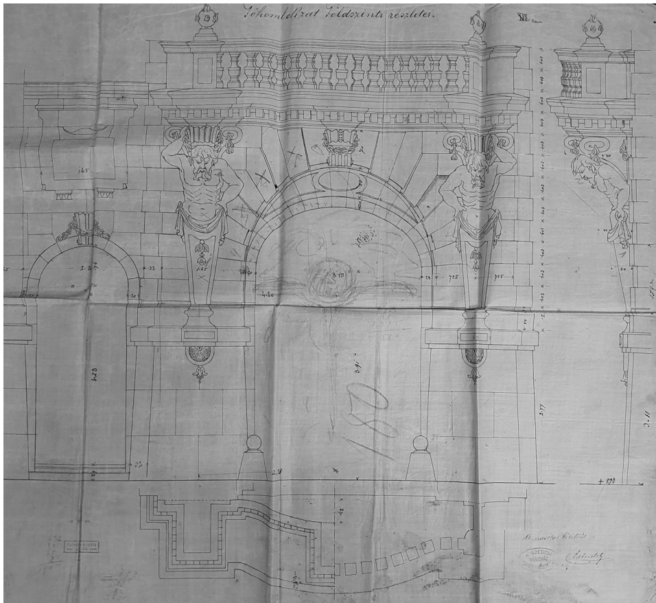
Lechner Ödön: A főhomlokzat földszinti részletei, 1882, mérnökpapír, 57×105 cm, MNL CSML, XV.2.b.47.180.
